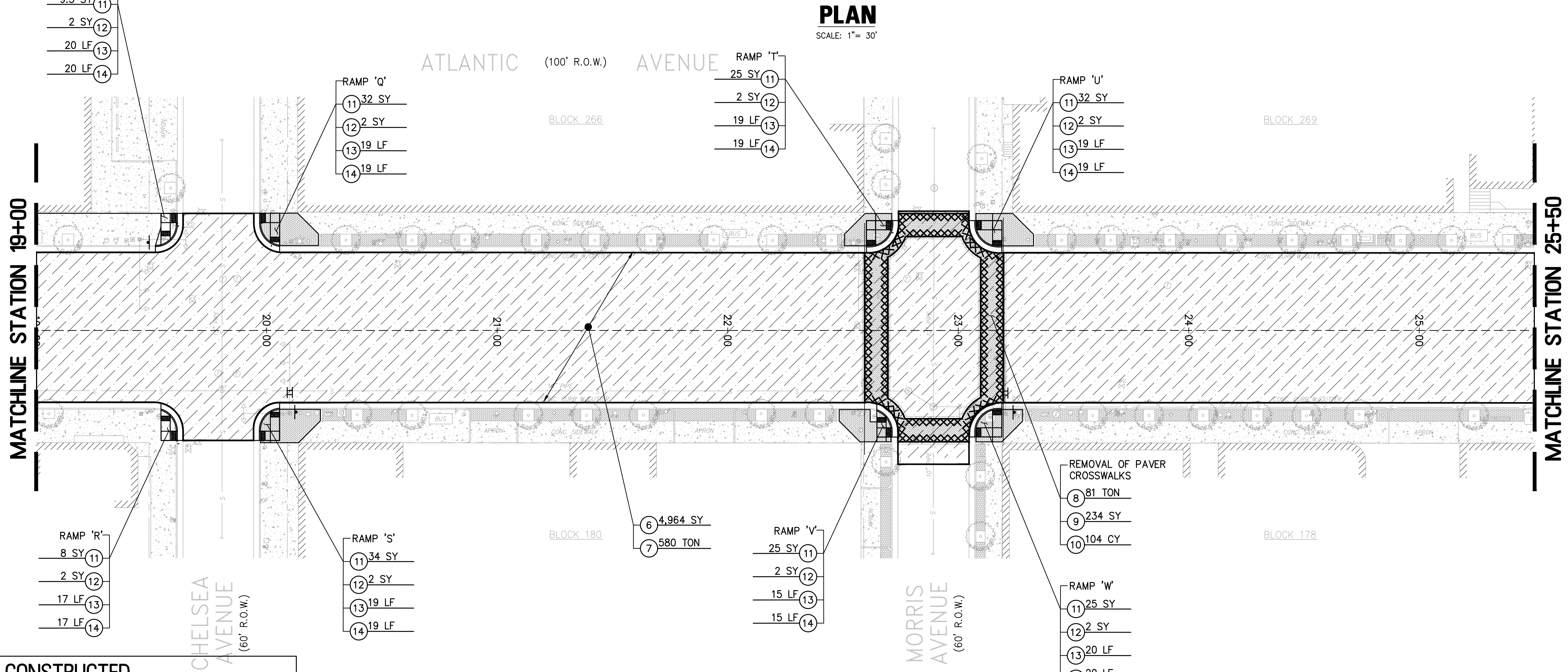
PLAN SCALE: 1" = 30'
