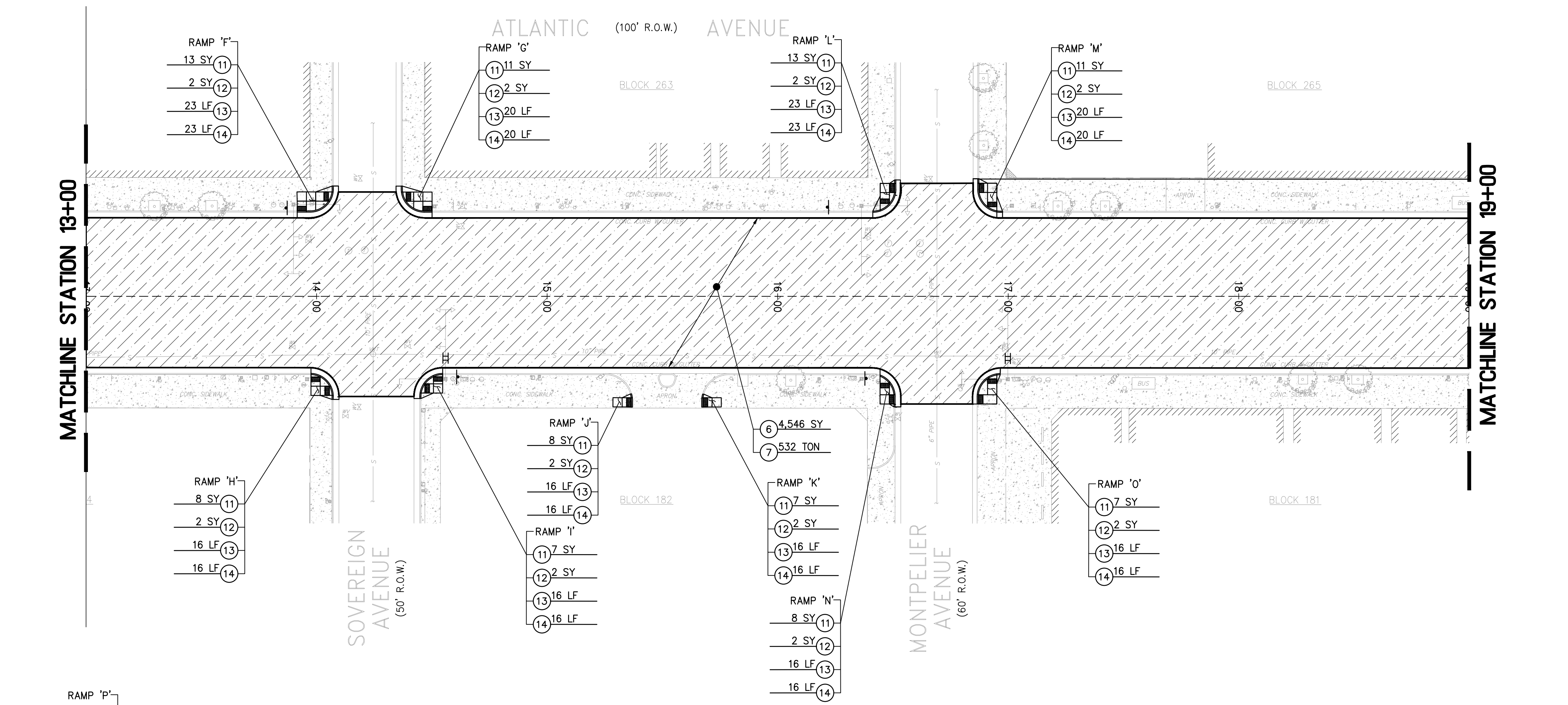
PLAN SCALE: 1" = 30'
