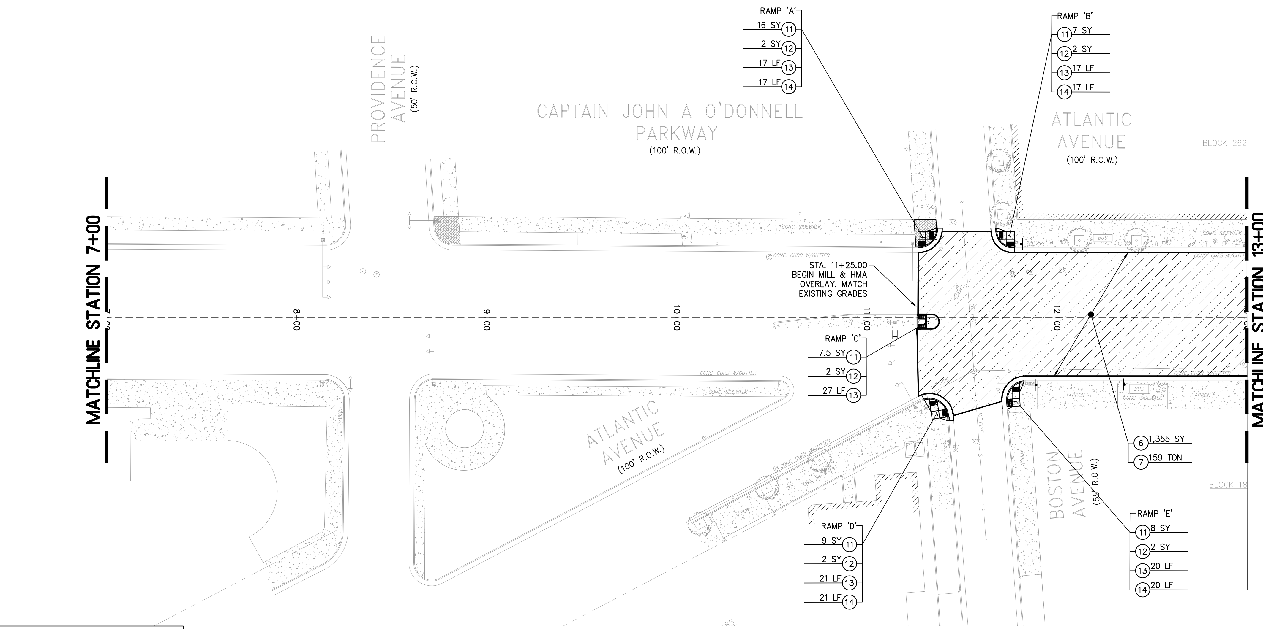
PLAN SCALE: 1" = 30'
